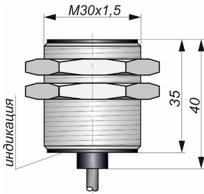
Габаритный чертеж
